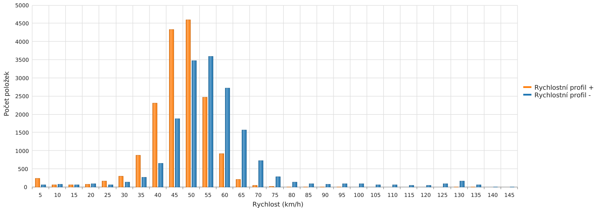
Ulice Těšov, Směr Mokřina, 50 km/h povolená rychlost Počet položek vs. rychlost
